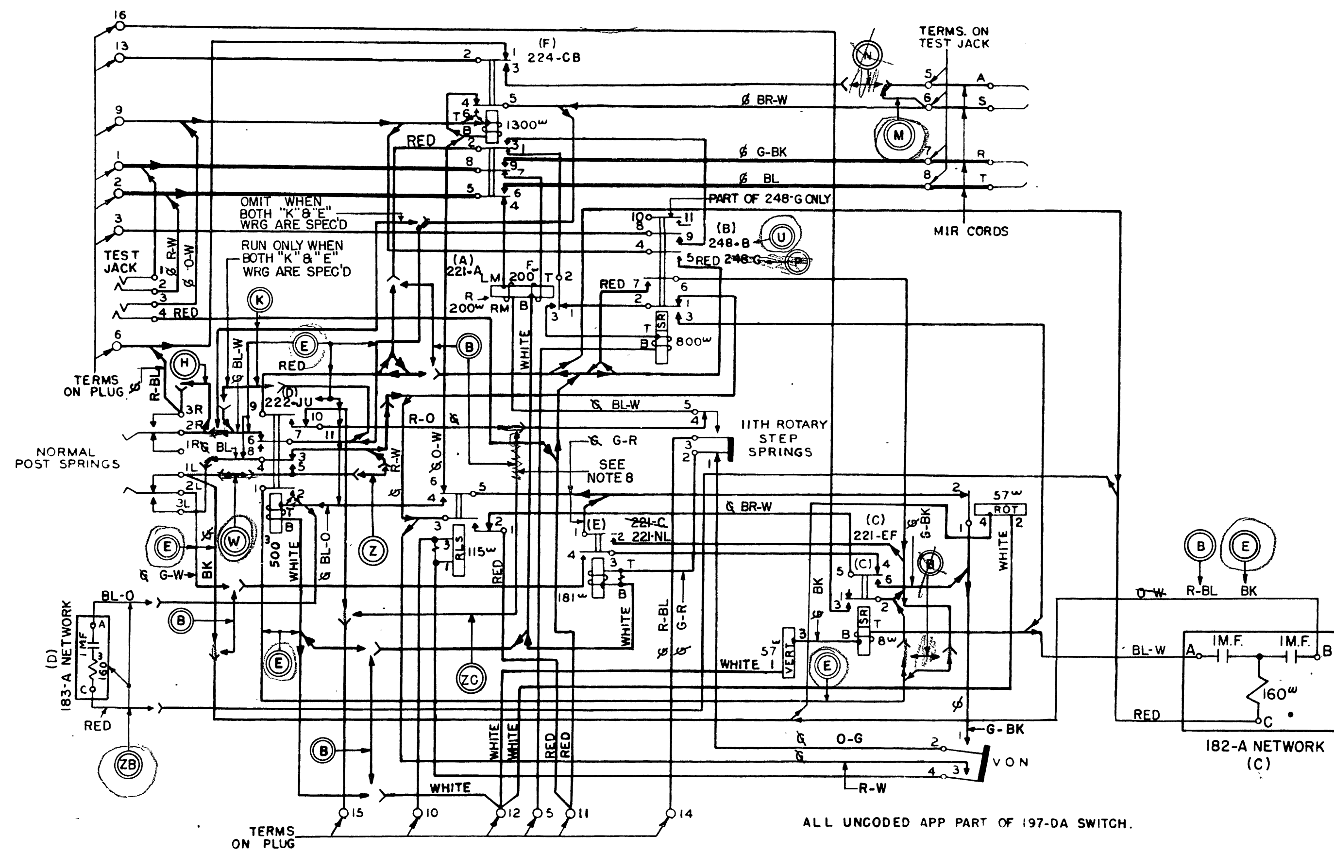
SELECTOR CKT.
